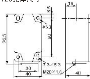
LXP1-120壳体尺寸
